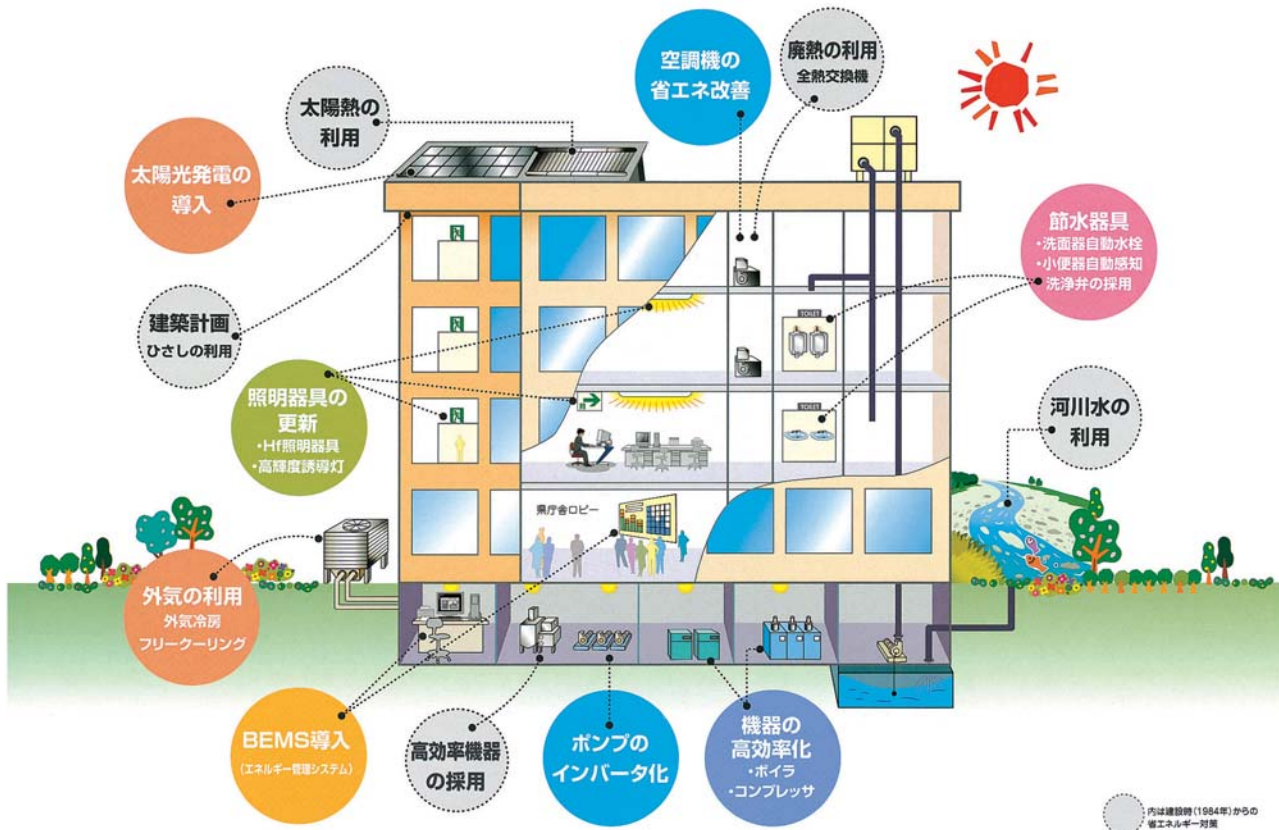
[山口県庁舎にみる省エネルギー化設備・手法]
