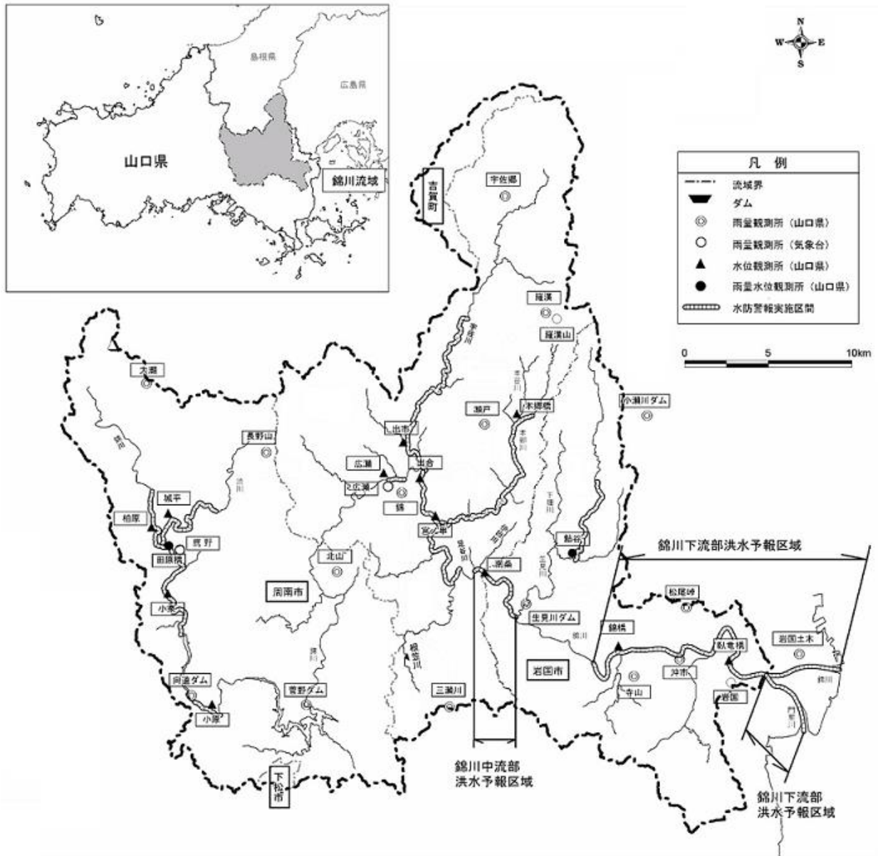
付図1 雨量・水位観測所配置図
