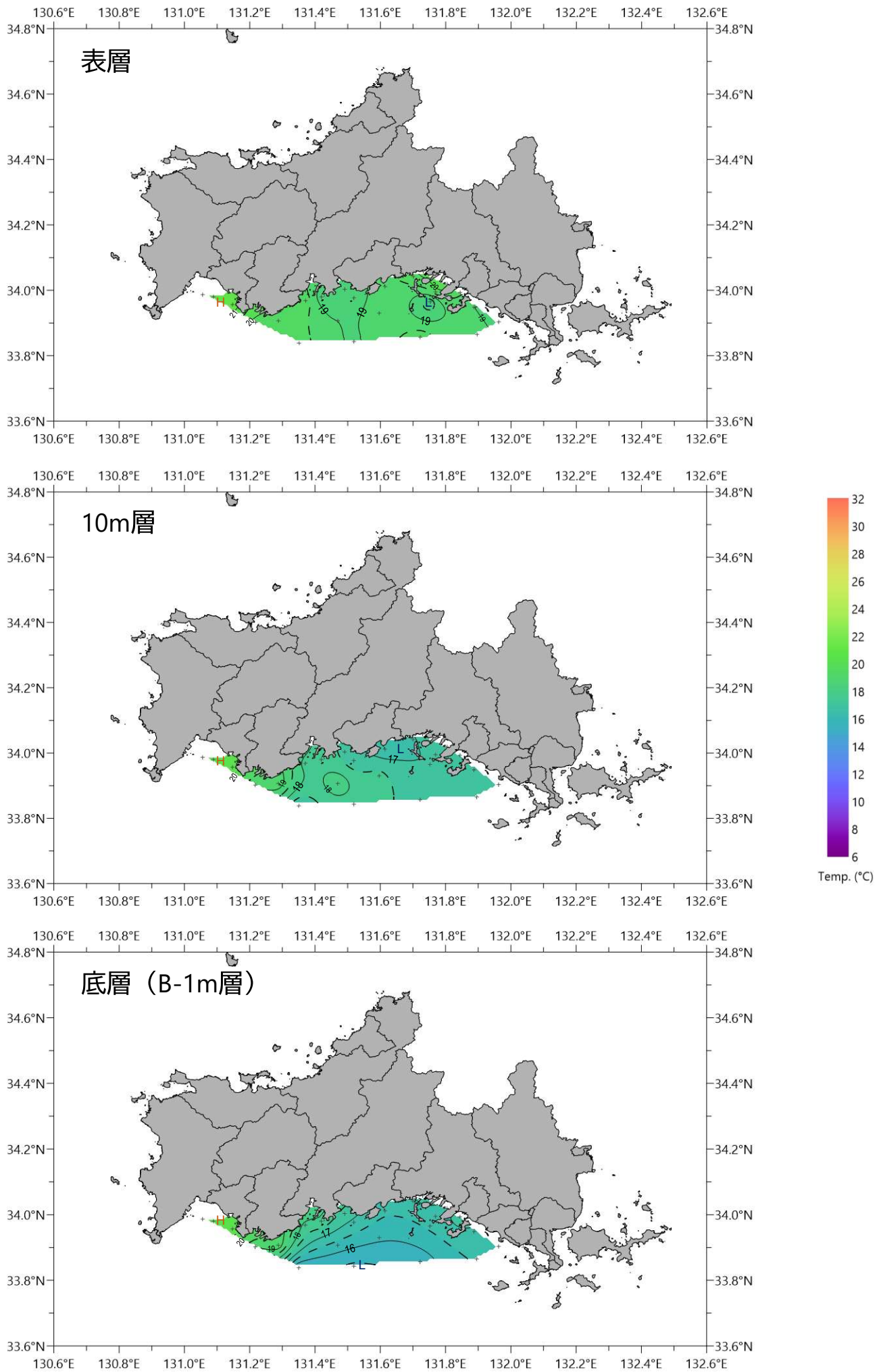
図. 水温の水平分布図(2024年6月4日観測)
