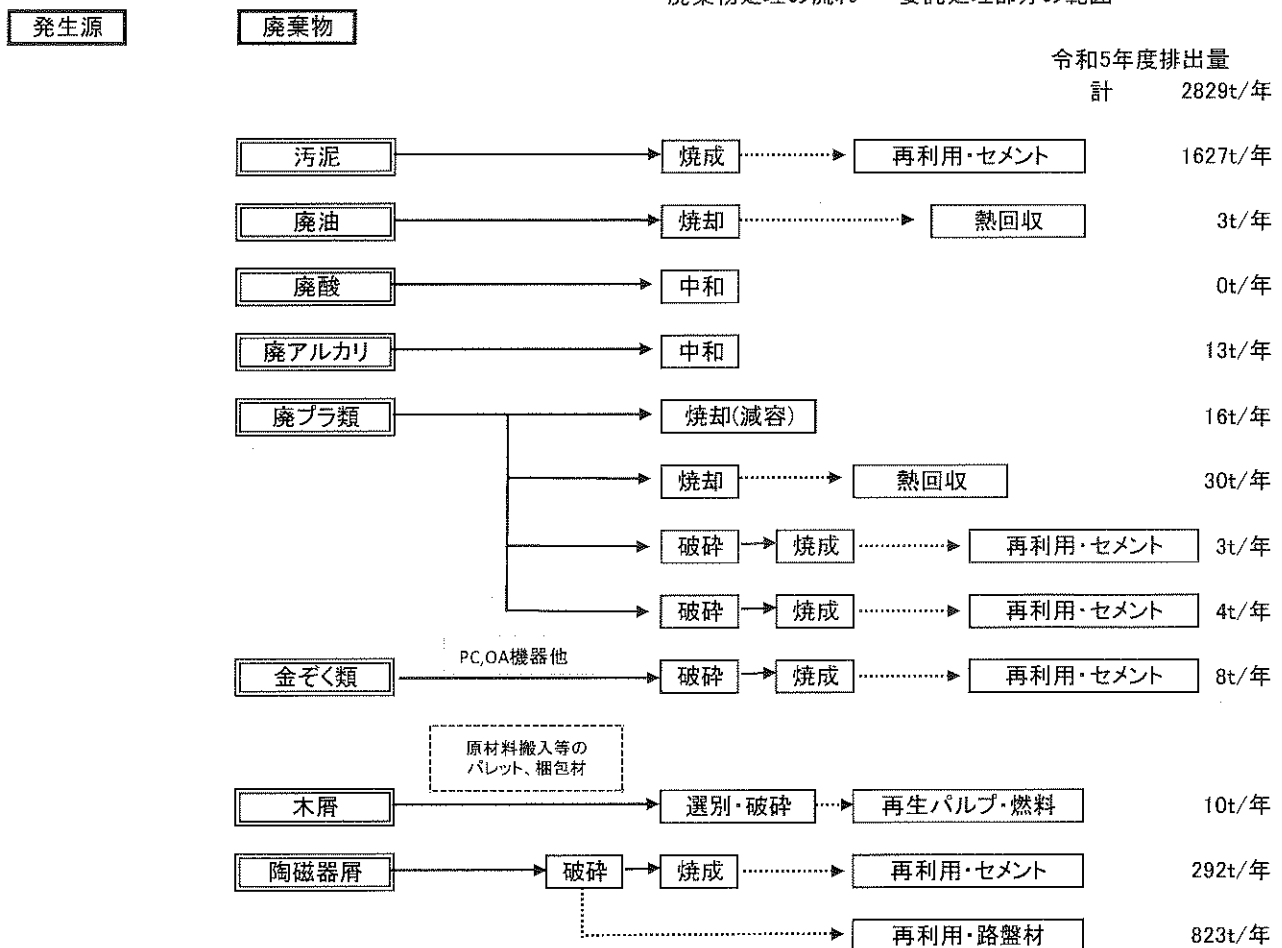
「図2」 廃棄物処理フロー図
