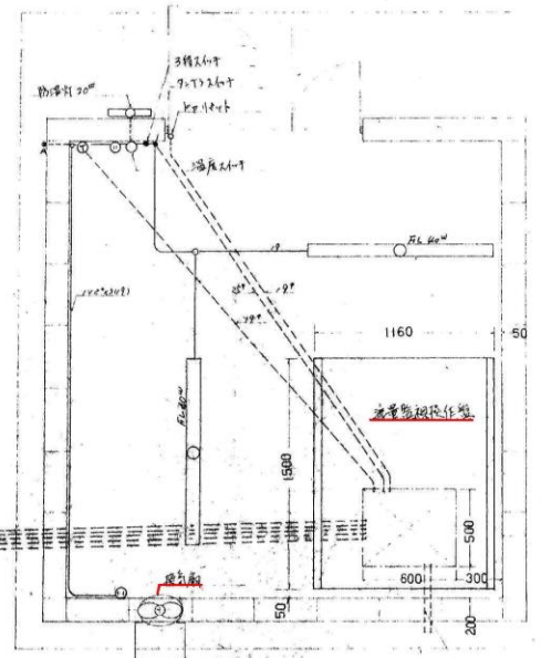
量水建屋平面図
