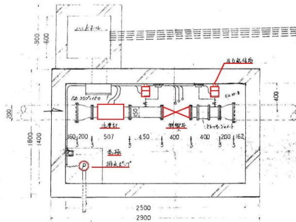
制御弁ピット平面図
