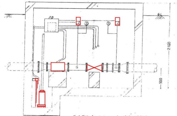
制御弁ピット断面図
