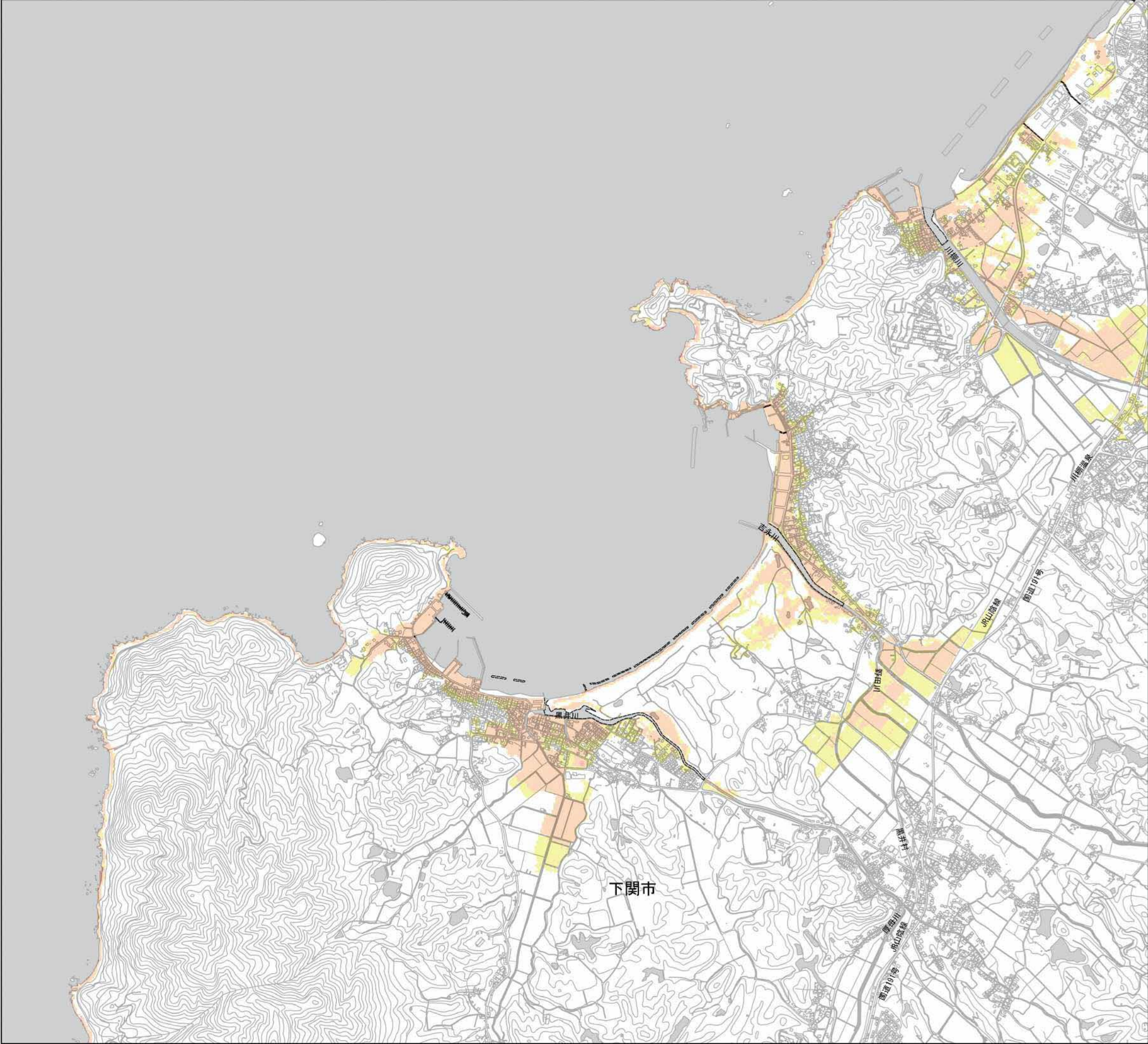
山口北沿岸 高潮浸水想定区域図 34 (浸水深)
