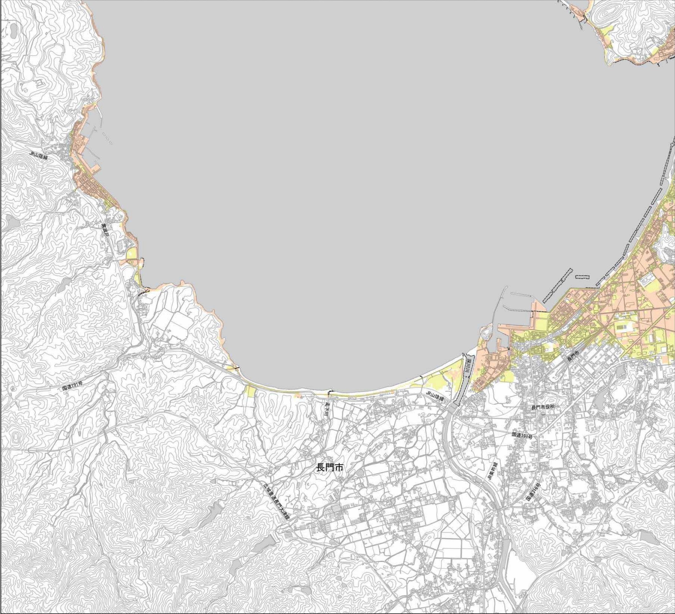
山口北沿岸 高潮浸水想定区域図 19 (浸水深)
