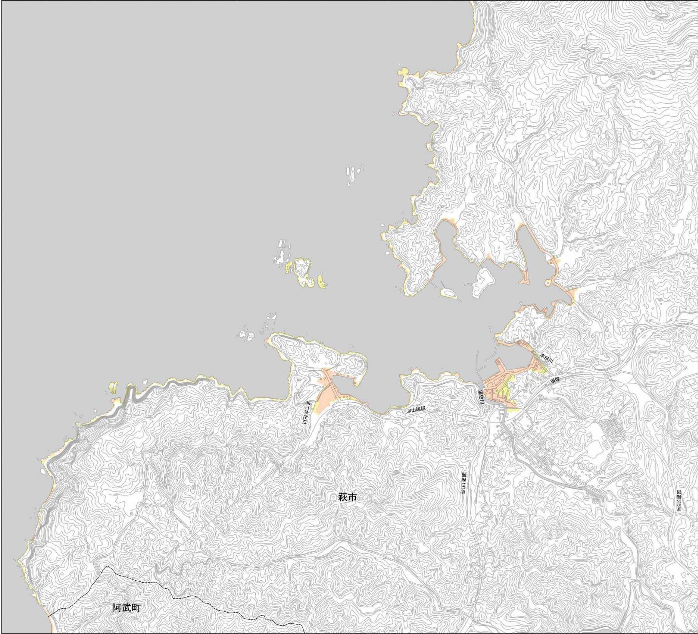
山口北沿岸 高潮浸水想定区域図 4（浸水深）
