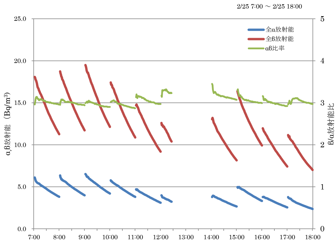
図4 全 \alpha ・ \beta 放射能の減衰(2月25日)
