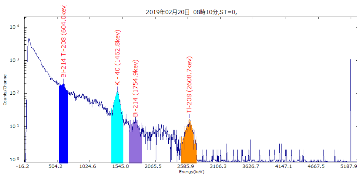
図2 平成31年2月20日 8:10 30.7nGy/h (最小値時のスペクトル)
