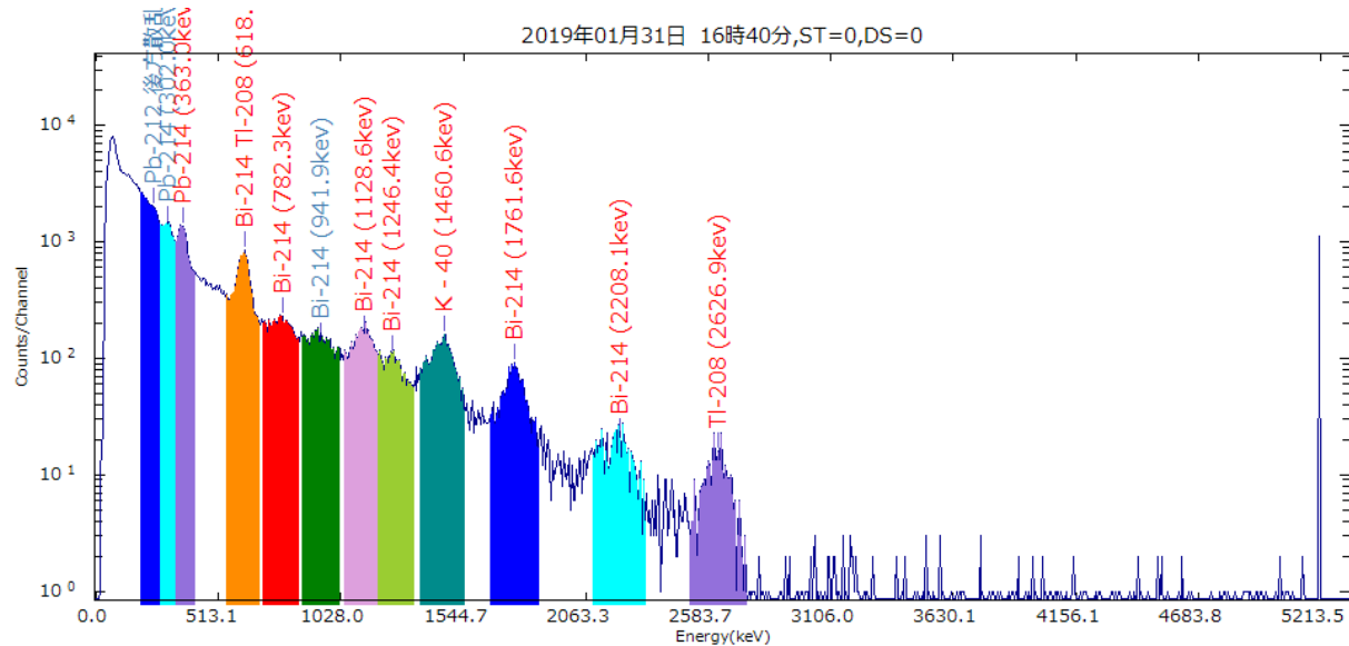
図1 平成31年1月31日 16:40 65.7nGy/h (最高値時のスペクトル)
