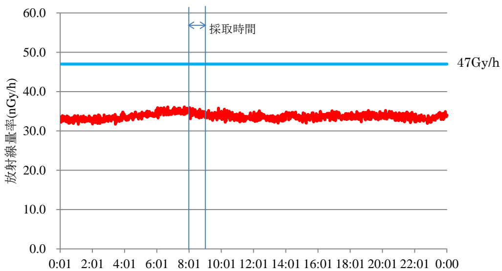
図5 空間放射線量率(2月25日)
