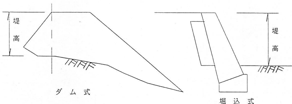
図5 堤高
