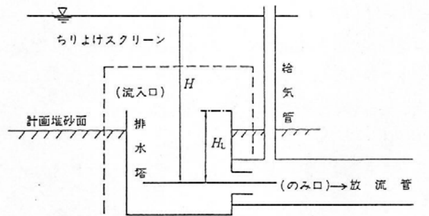
図11 放流施設流入部構造
