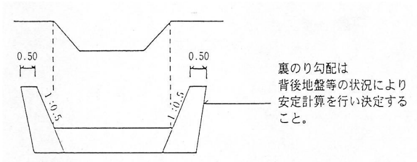
図13 側壁護岸と洪水吐等
