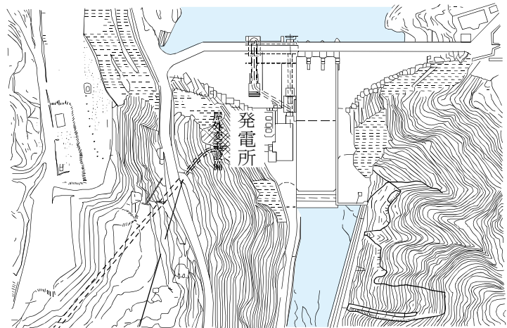
菅野ダム、発電所平面図
