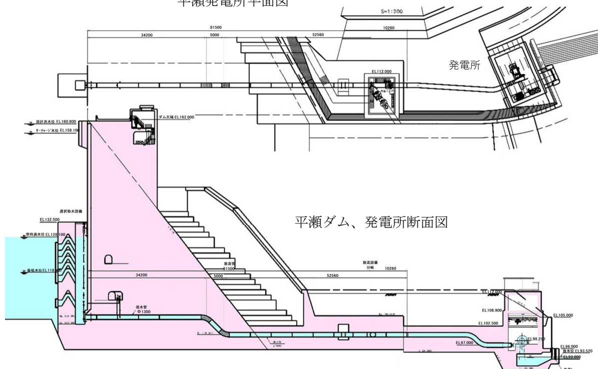
平瀬発電所平面図
