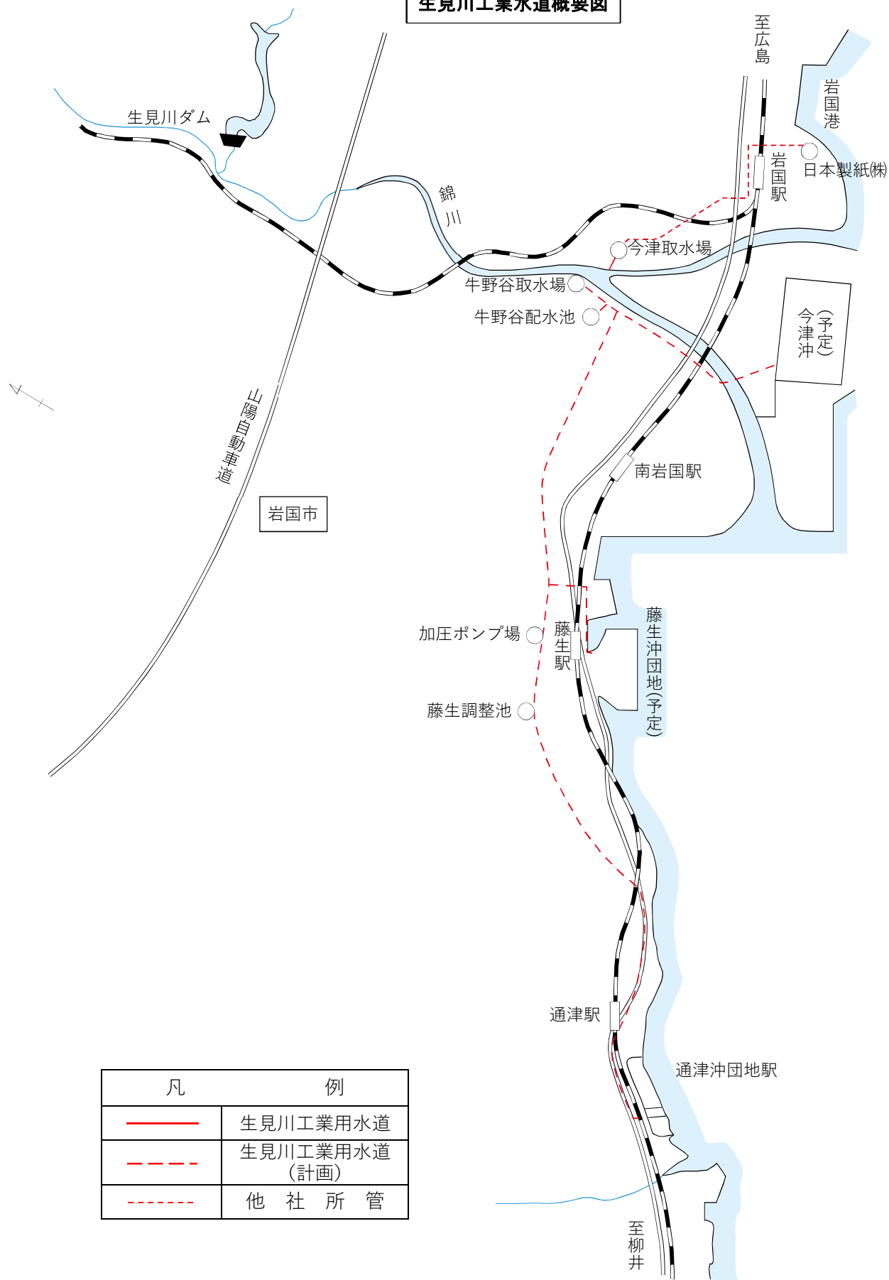
生見川工業水道概要図
