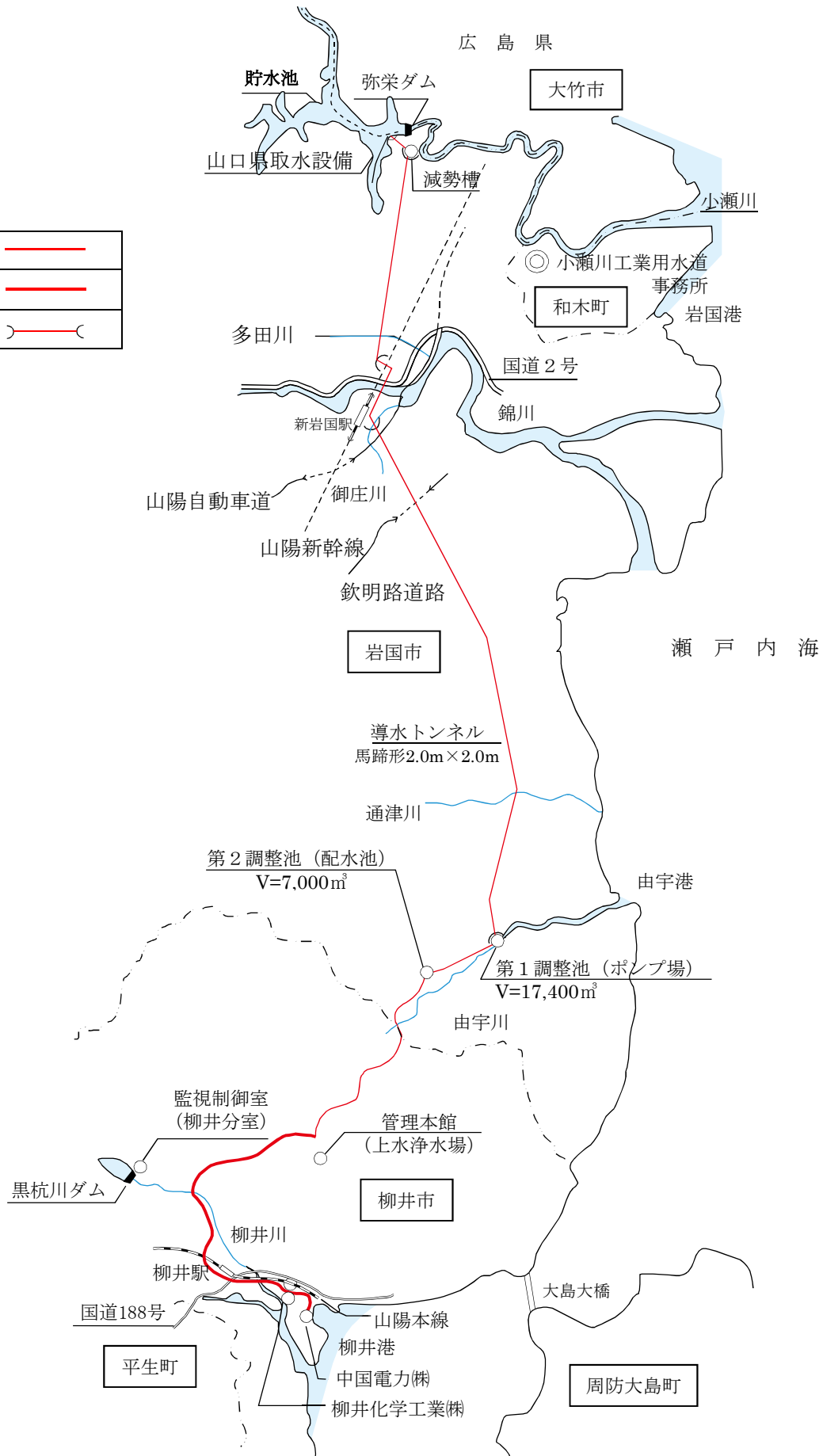
小瀬川第2期工業用水道概要図
