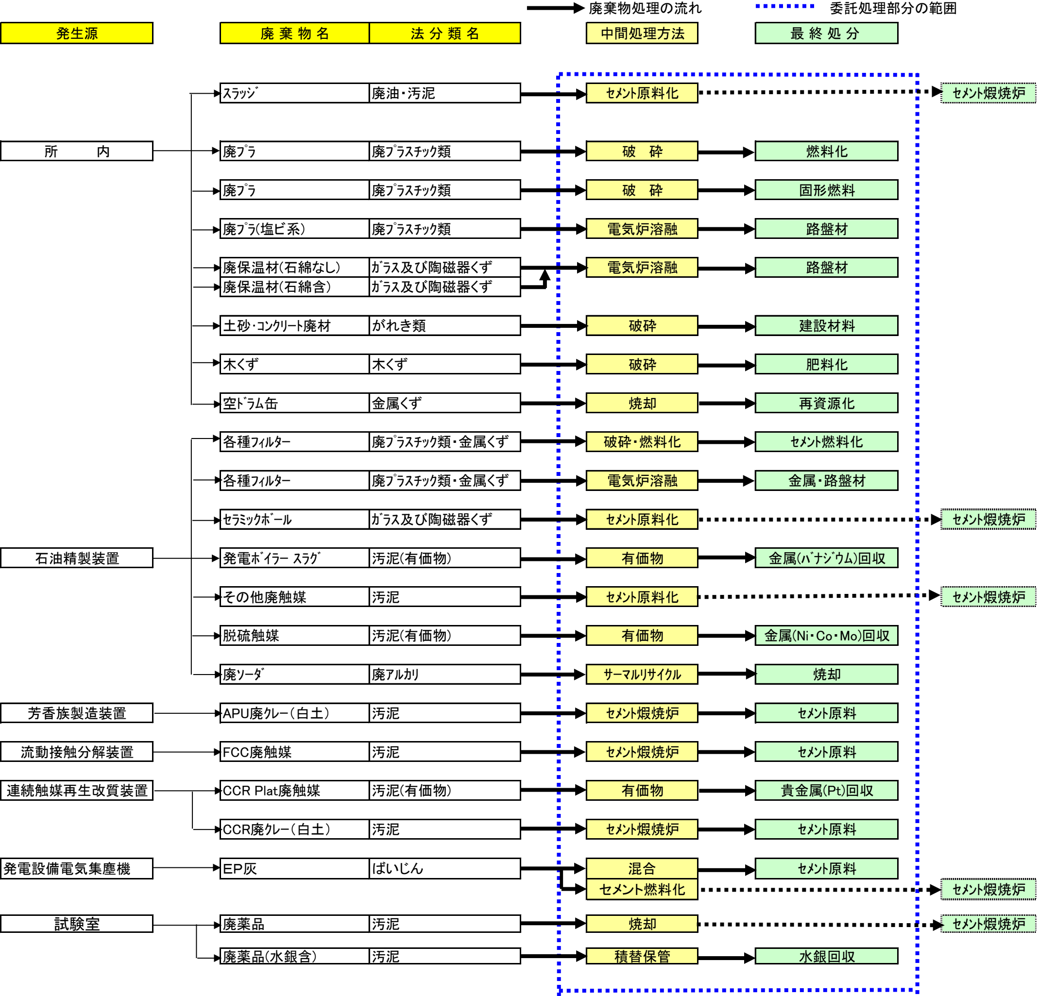
<別紙1-1> 廃棄物処理フロー図
