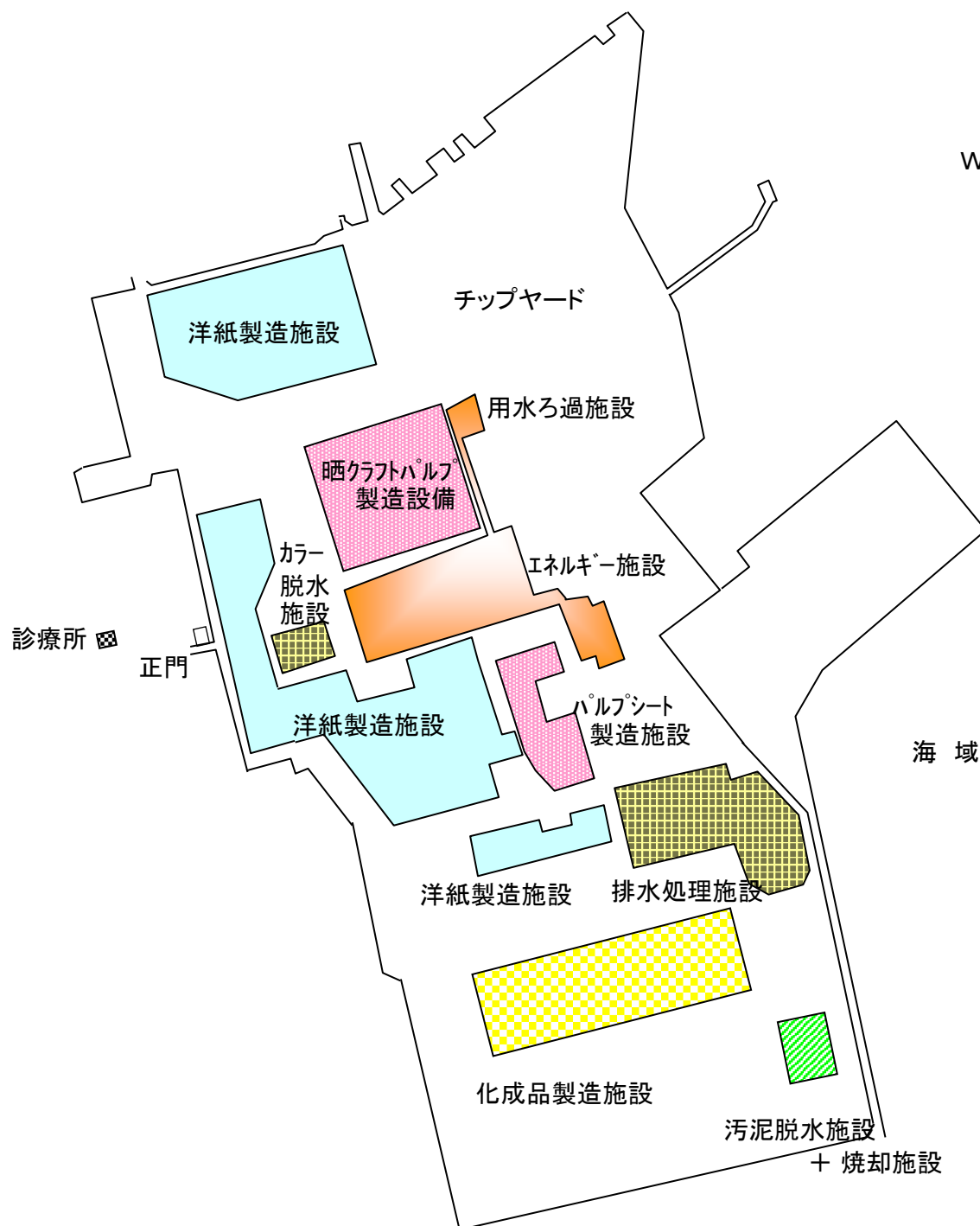
図-1 工場配置図
