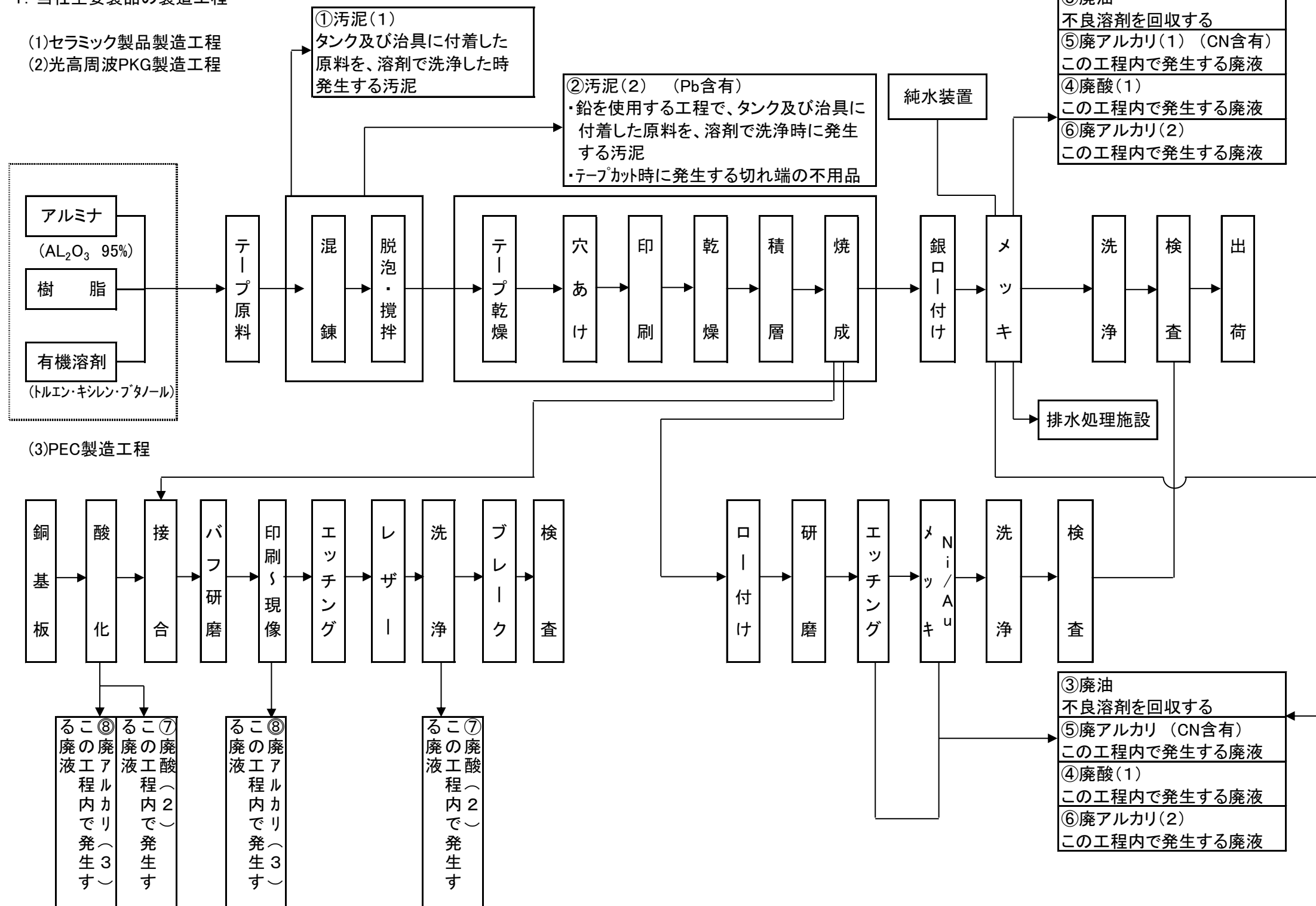
製造工程フロー図及び特別管理産業廃棄物発生フロー図－1
