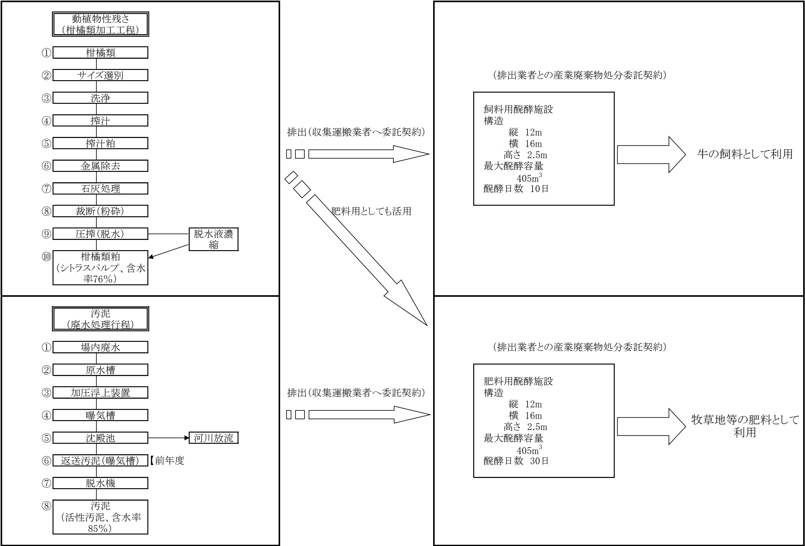
図1: 動植物性残さ、汚泥等の処理工程図 日本果実工業株式会社萩工場
