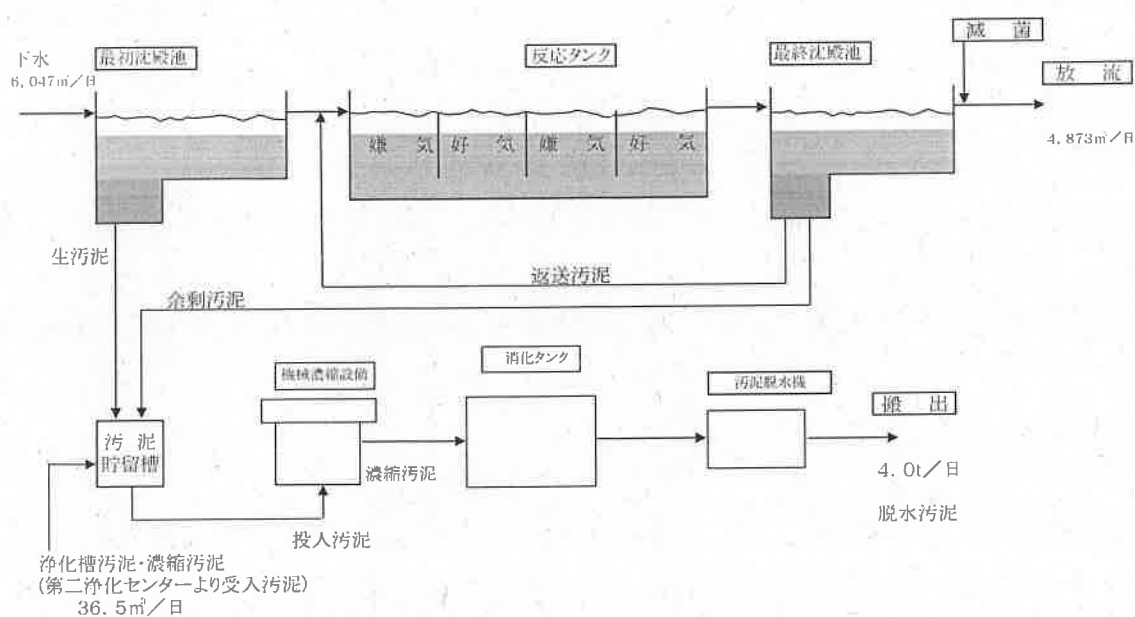
図1 萩浄化センターフローシート (流量等は6年度平均)
