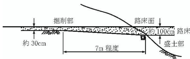
図2-3 掘削（切土）部、盛土部接続部のすり付け
