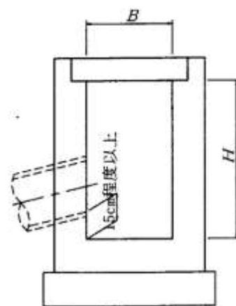
図-6 泥だめ
