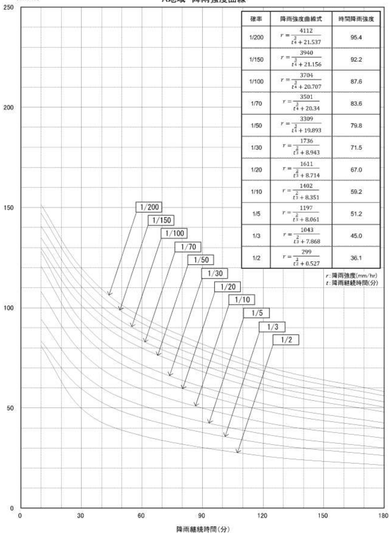
A地域 降雨強度曲線
