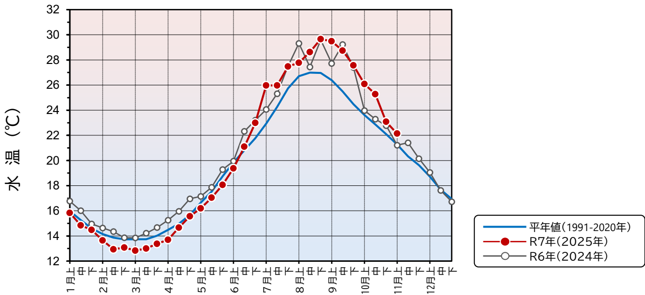
図. 萩沖北北西15海里における表層水温(旬ごとの平均値)の推移
