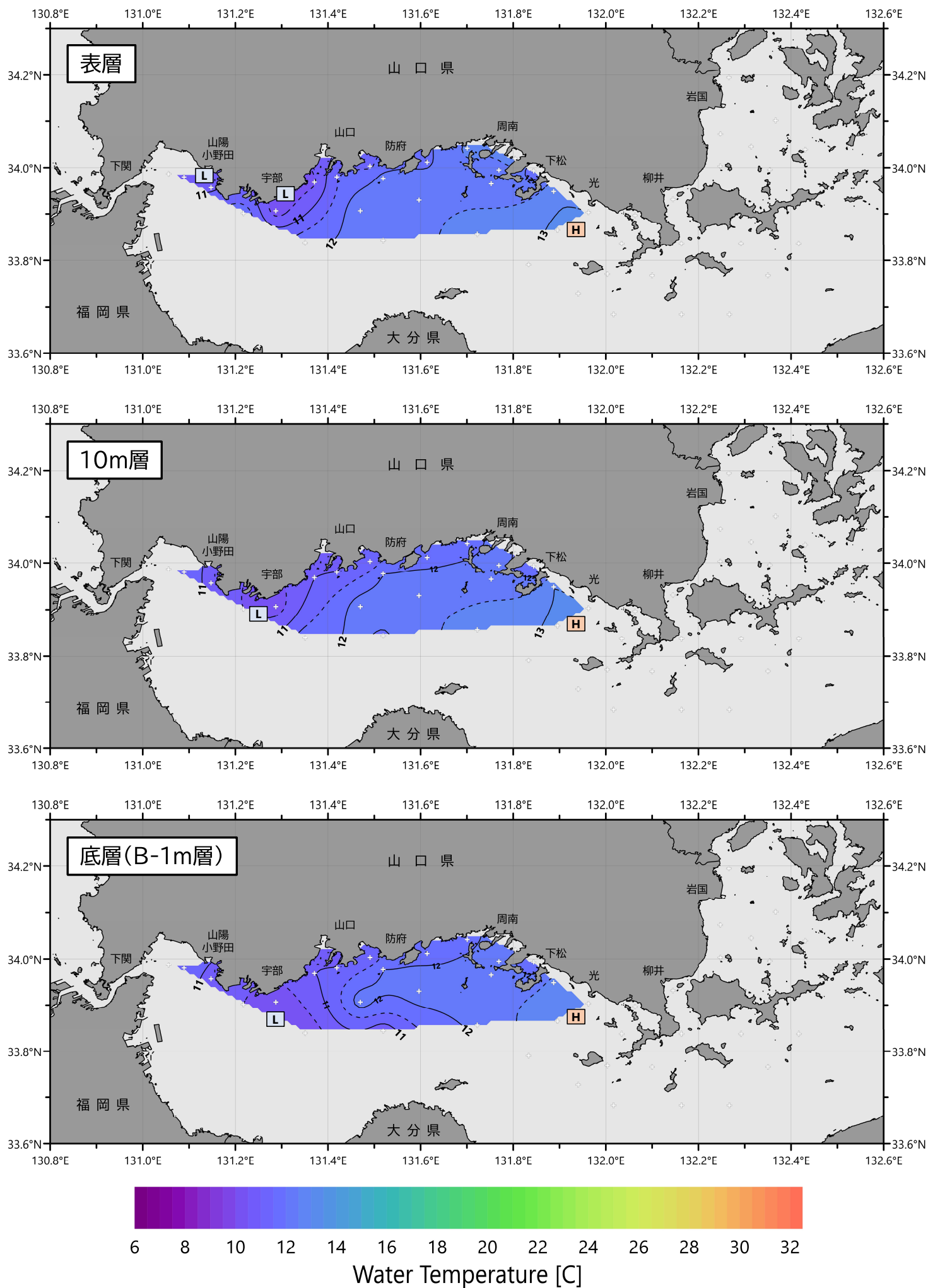
図. 水温の水平分布図 (2026年1月17日観測)
