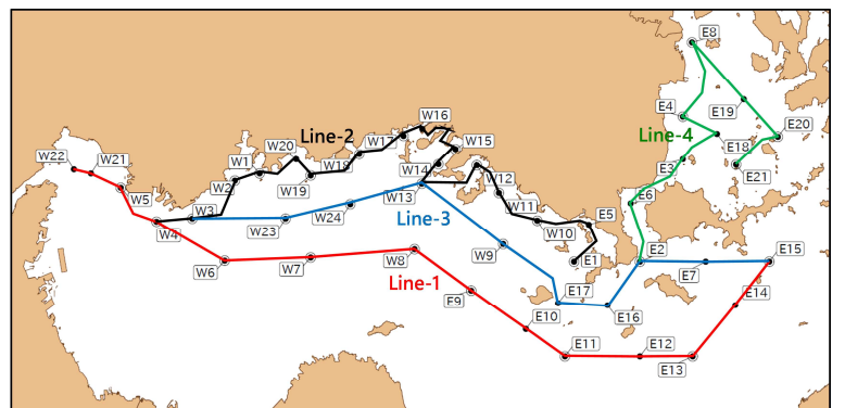
図. 水温の鉛直断面図 (2026年5月7・11・12日観測)
