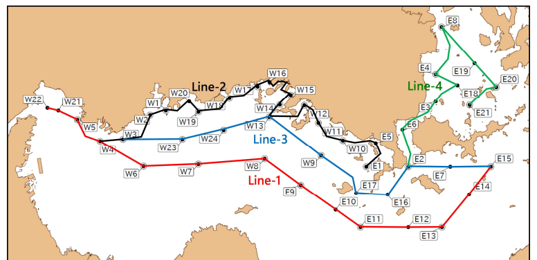
図. 水温の鉛直断面図 (2026年7月3日観測)
