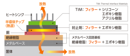
半導体における放熱材の使用部位
