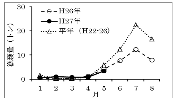
山口県代表 2 地区のイカ釣りによるケンサキイカ漁獲量
