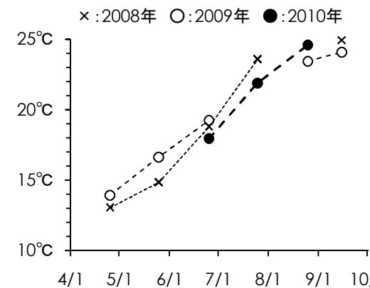
図. 7調査点における平均水温(10m層)の推移(2008~2010年の4~9月)
