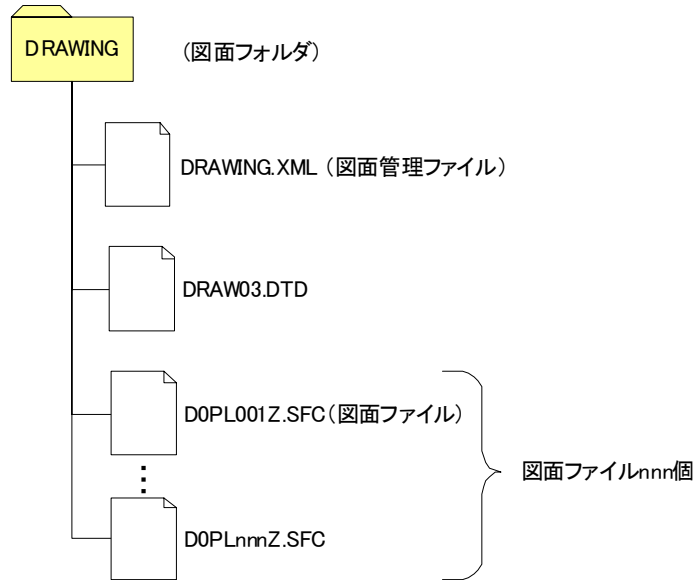
図 2-5 図面ファイルのフォルダ構成
