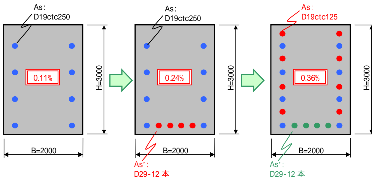
図 3.2.32 補強鉄筋配置例
