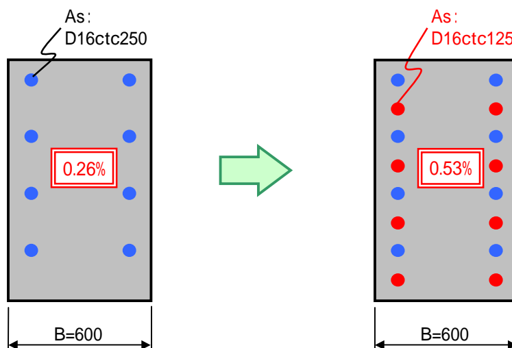
図 3.2.36 補強鉄筋配置例
