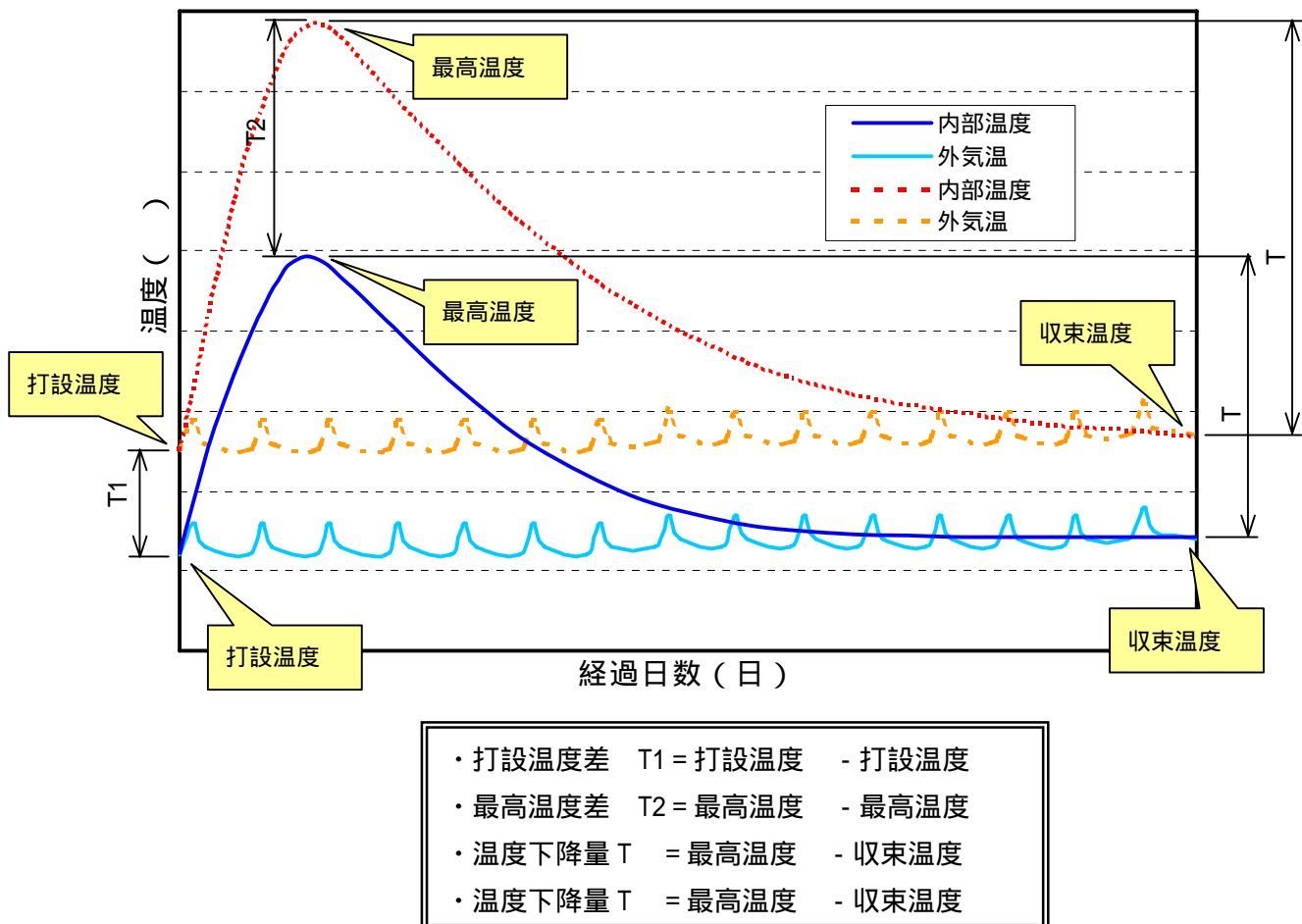
図 2.2.1 コンクリート内部温度の経時変化
