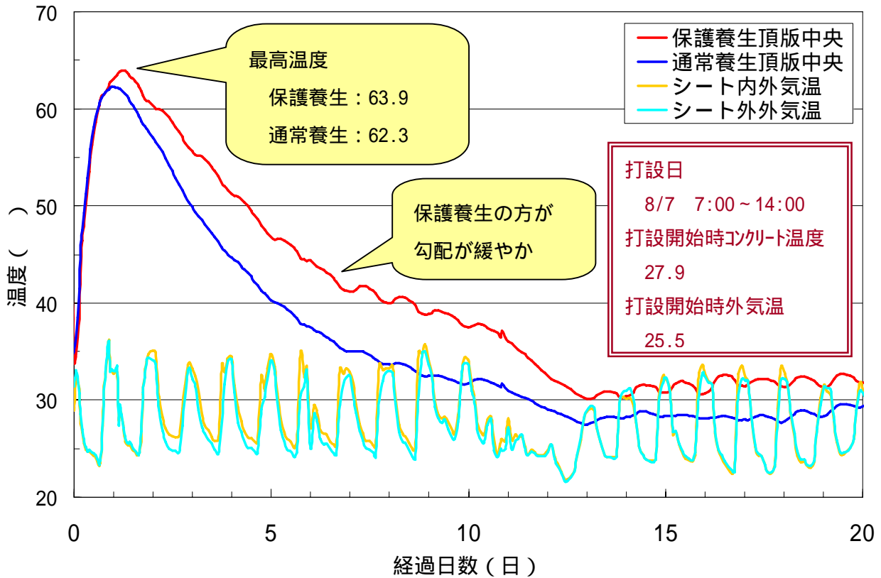
図 3.4.3 温度計測結果 (頂版中央)
