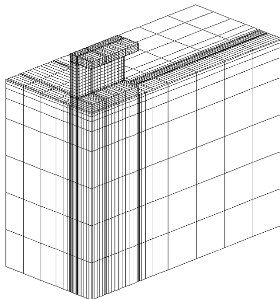
図 3.3.5 解析モデル全体図 (1/4 モデル)
