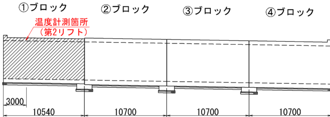
側面図
