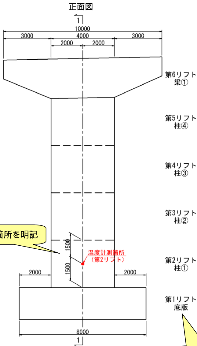
打設リフト図
