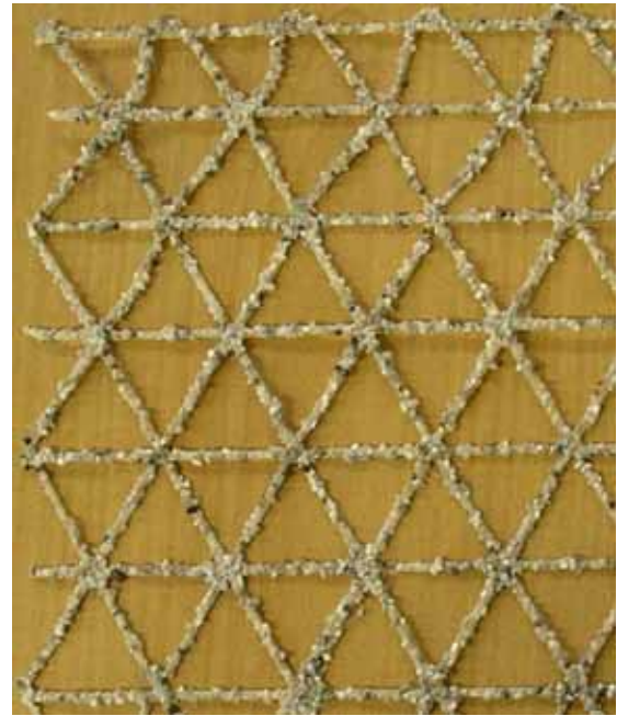
図 3.2.2 アラミド繊維拡大写真
