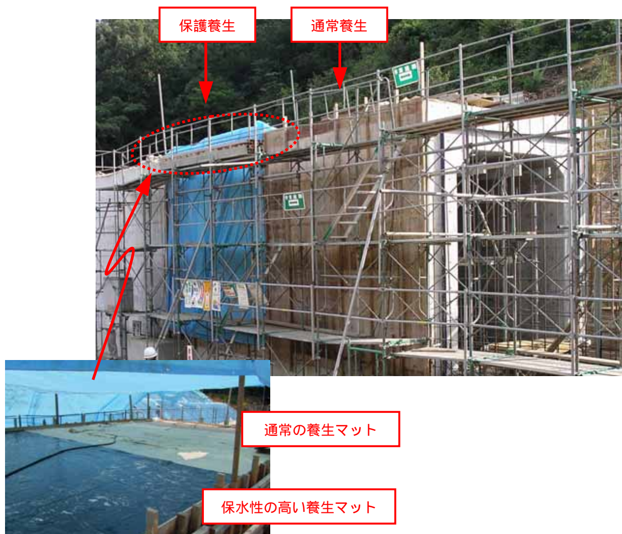
図 3.4.2 養生効果確認実施状況（H18 試行施工）
