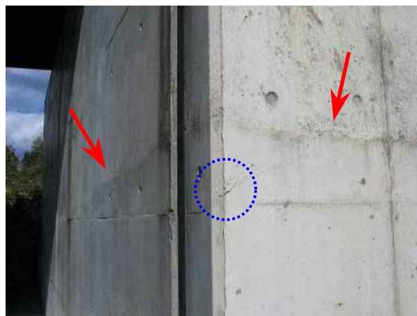
○は沈下ひび割れ 【橋台たて壁】
