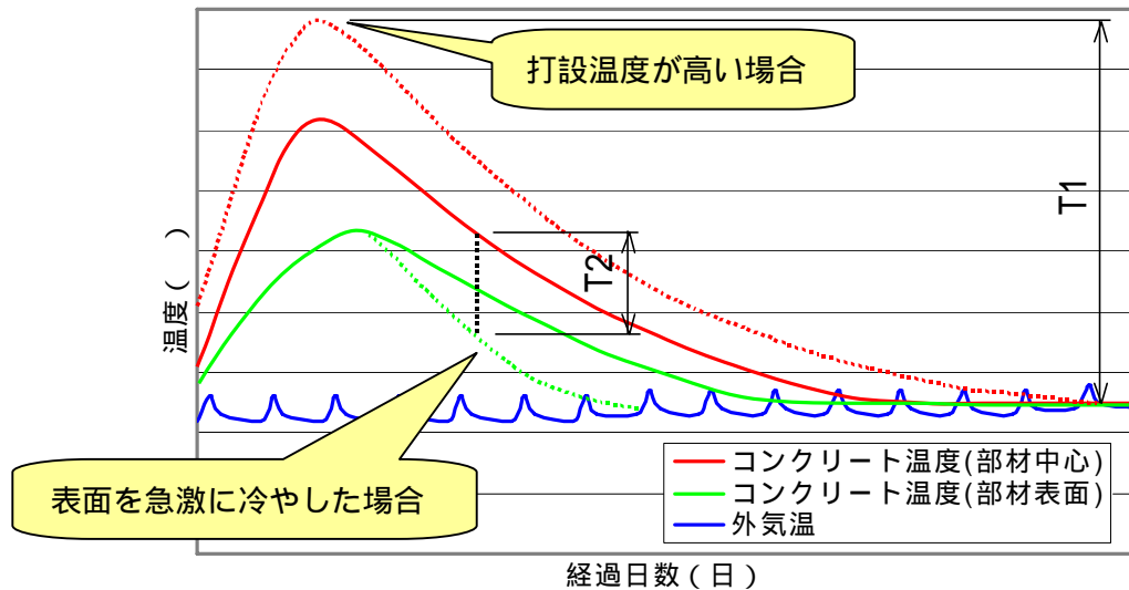
図 5.3.1 コンクリートの内外温度と外気温
