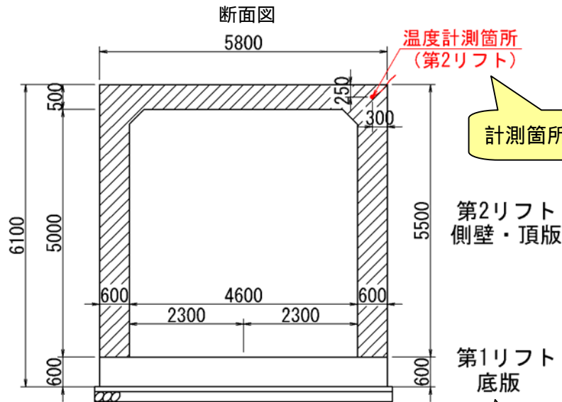
打設リフト図
