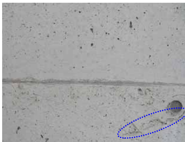
○ は沈下ひび割れ 【左写真の拡大】
