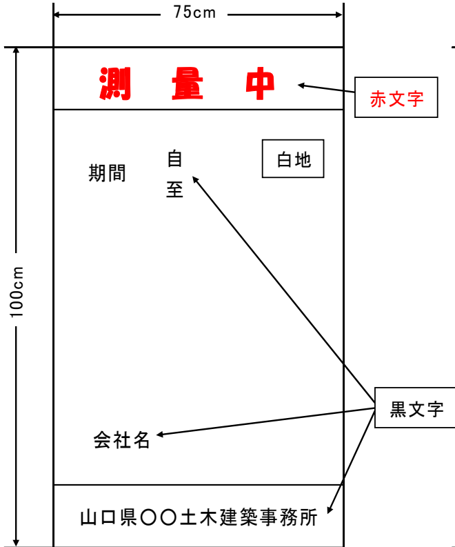
①案内表示板
