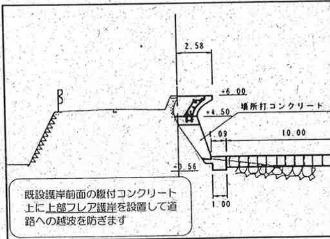
護岸断面図
