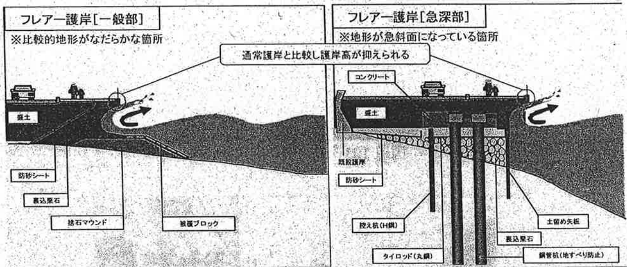
▲フレア護岸の構造図
