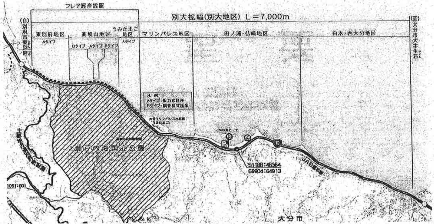
▲別大拡幅 平面図
