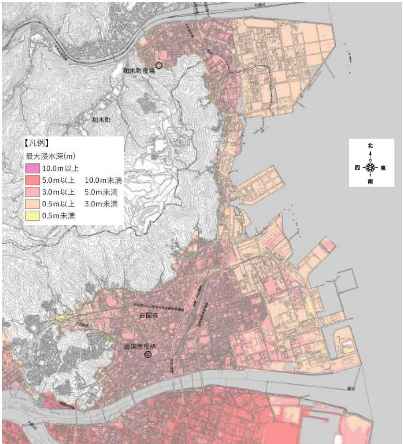
図3-2 岩国市・和木町の高潮浸水想定区域図
