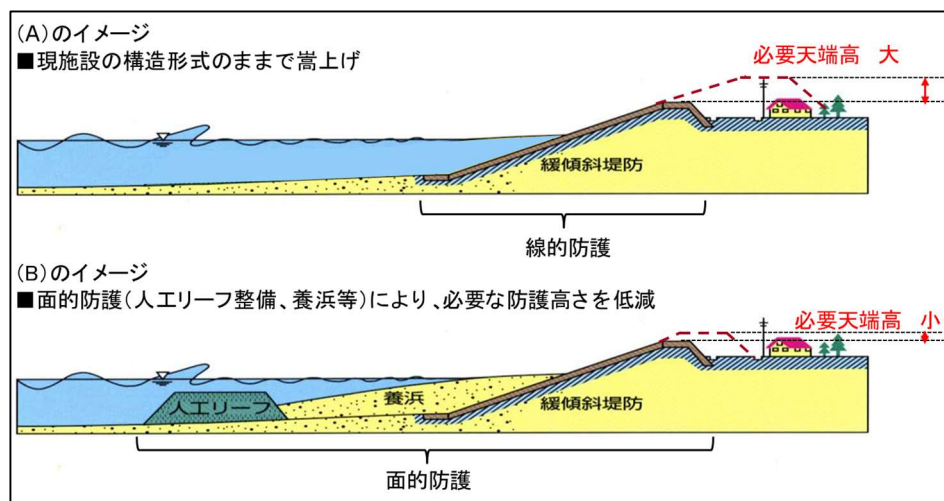
図－7 線的防護・面的防護による必要天端高のイメージ
